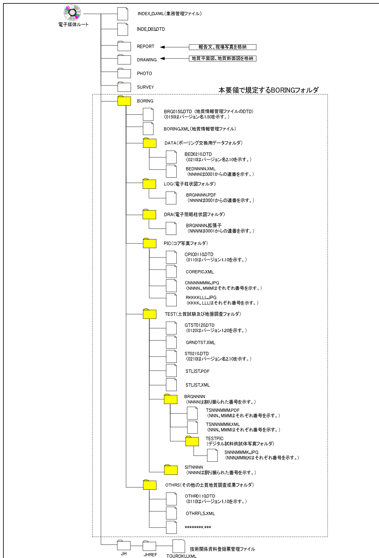
図 3-1 フォルダ構成
