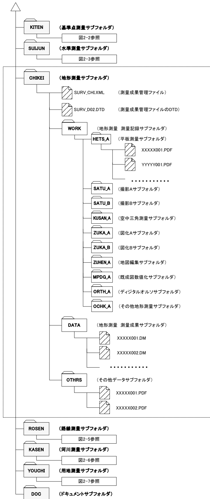
図2-4 「CHIKAI」フォルダ内のサブフォルダ構成
