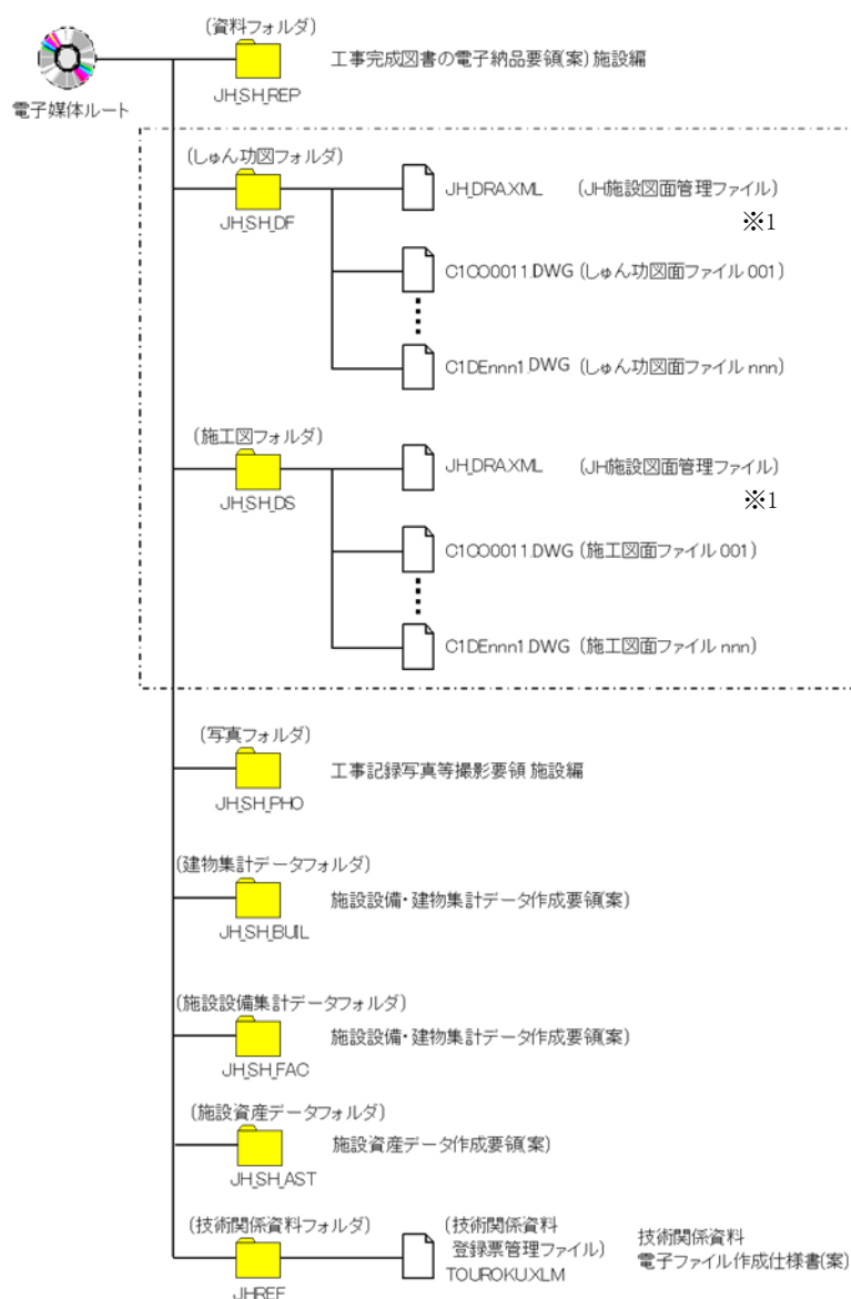
図 3-3-2 「施設工事完成図書の電子納品要領(案)」のフォルダ構成
