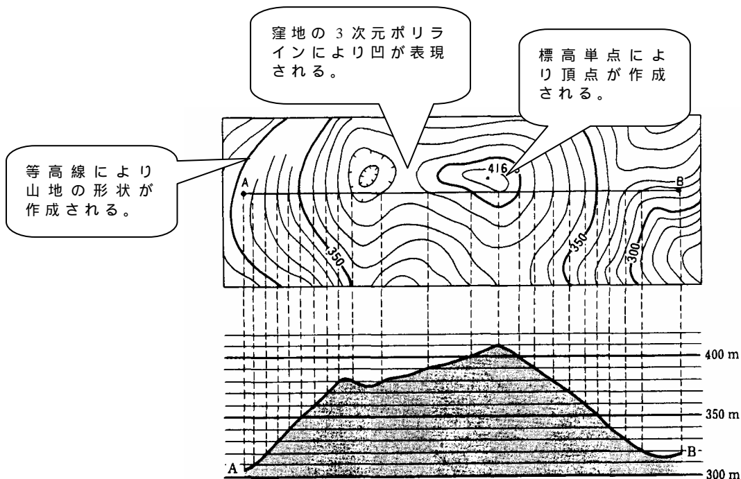
図 2-1 地形形状の抽出
