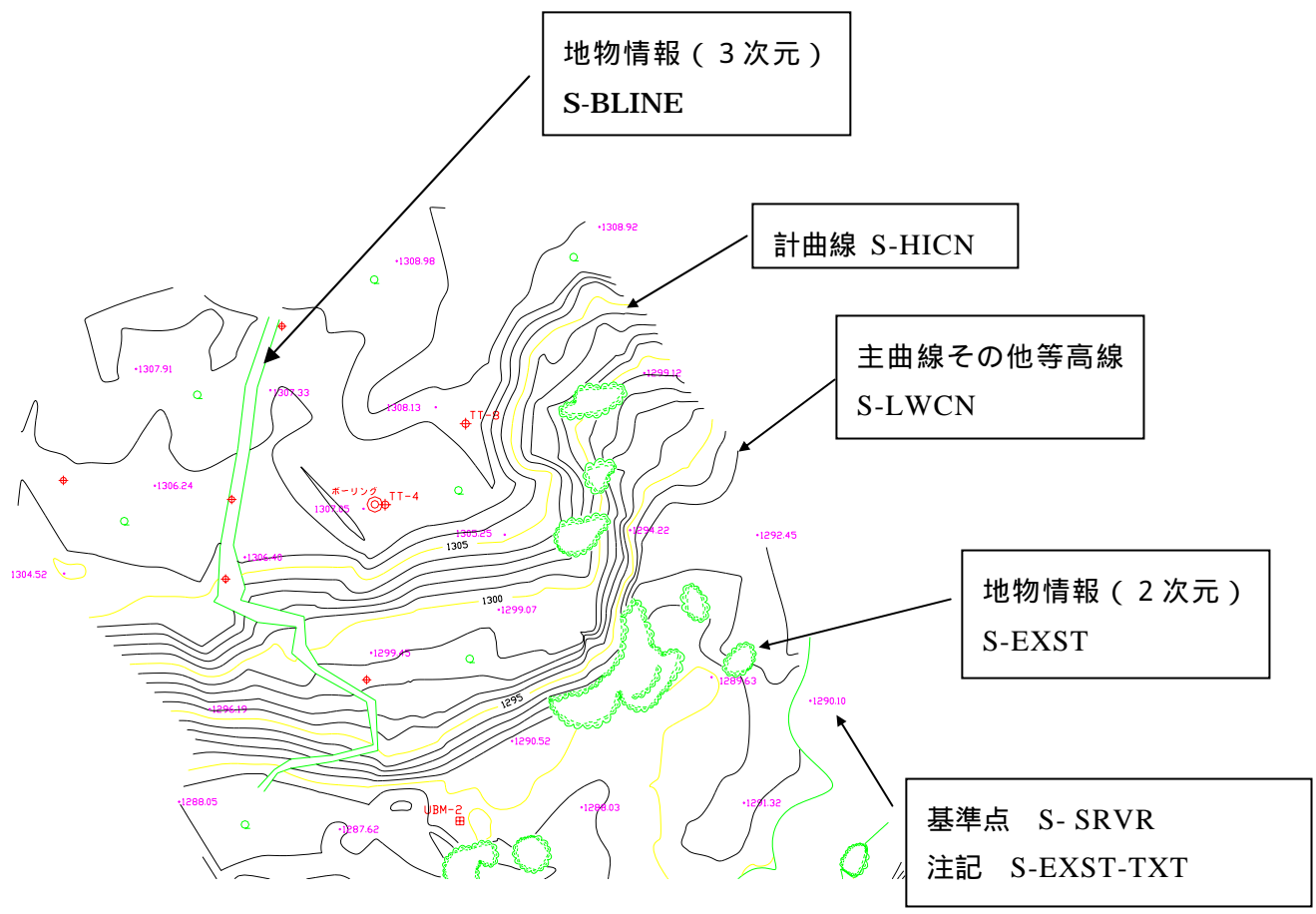
図 2-2 レイヤ名設定の例
